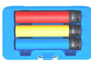
BGS74567 1/2 17-19-21mm Voor alu velgen-jantes alu L=150mm
